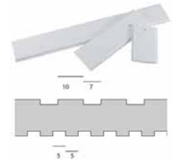
PDS34. Скребок фигурный двусторонний 17 см. Размер резиновых зубцов с одной стороны 10x7 мм, с другой- 5x5 мм. Длина скребка 34 см.
