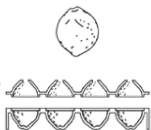
AF006. Набор ЛИМОН из двух частей; общий размер формы 300x175 мм; размер ячейки: Ø53 мм, h 70 мм, v 8 ячеек по 85 мл
